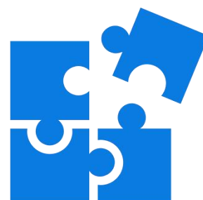
嵌入式支持
