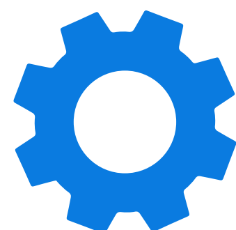
自定义主题
